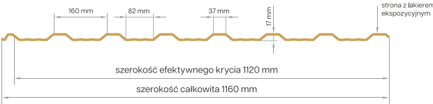
Profil dachowy
