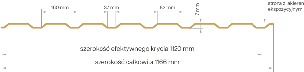
Profil elewacyjny
