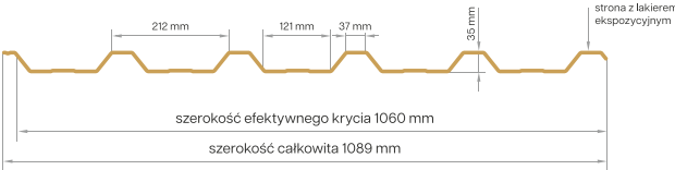
Profil dachowy
