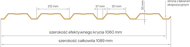
Profil elewacyjny
